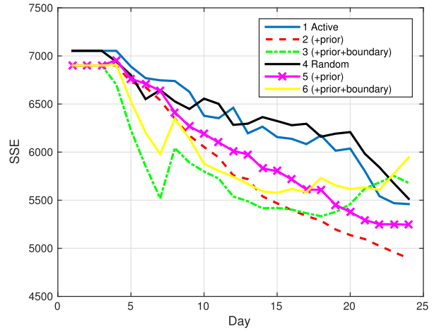
(d) User 4.
