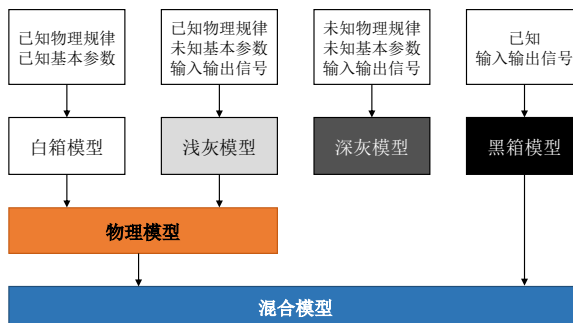
图 5 混合模型
